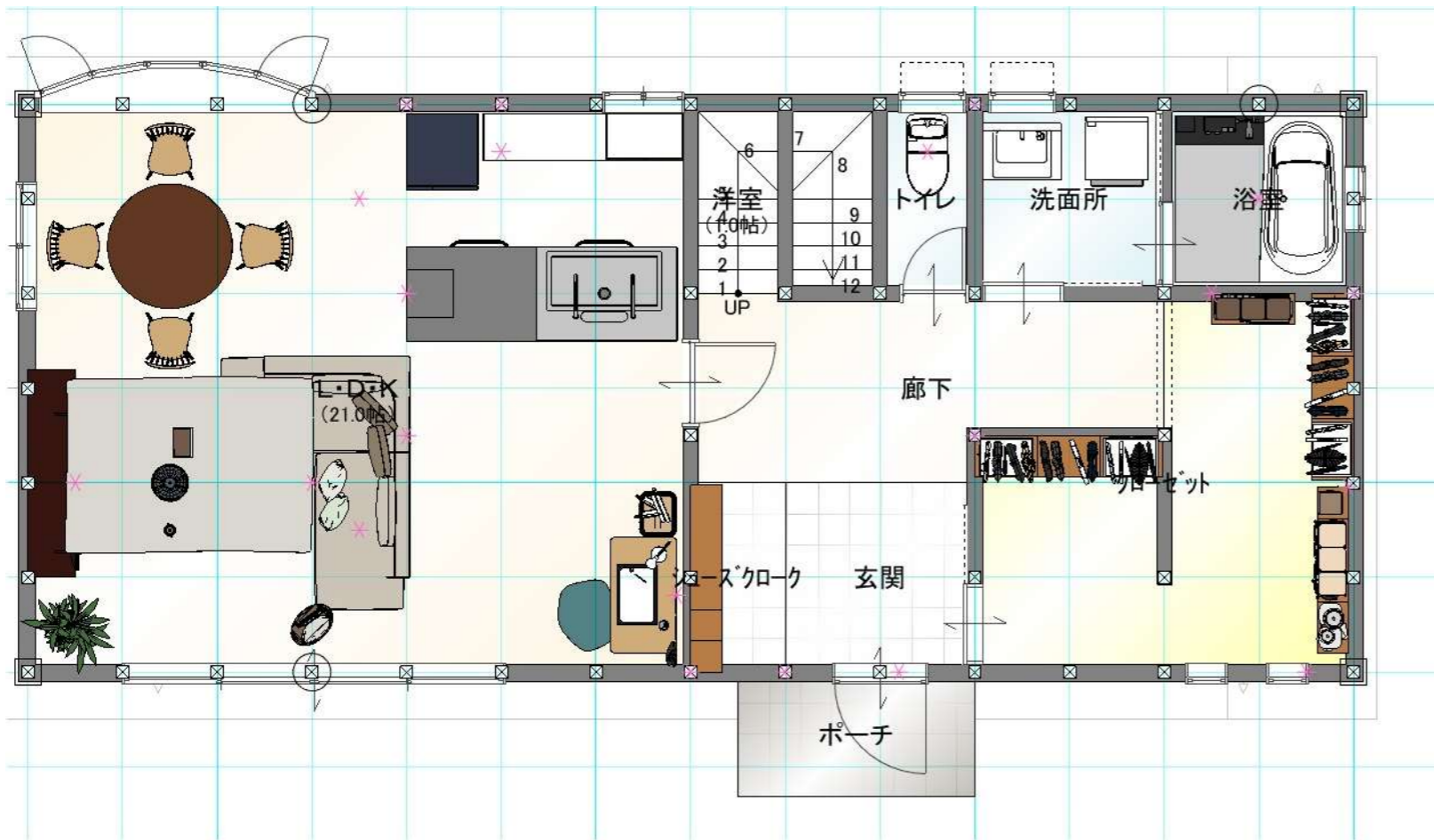
■ 1階平面図
